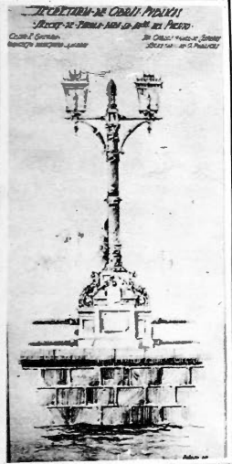
Una de las farolas que se situarán en la Avenida del Puerto. (Proyecto de César Guerra)
